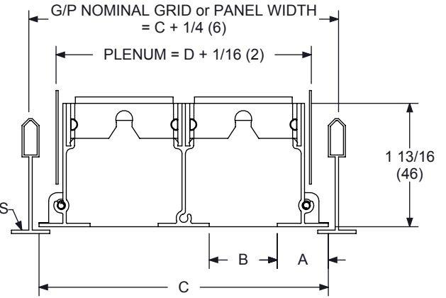
SECTION A-A NO BLADES
