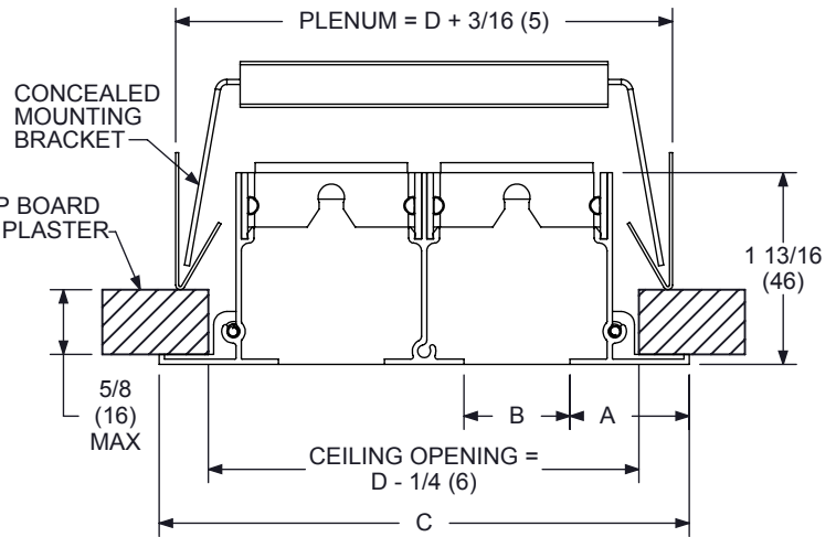
SECTION A-A NO BLADES
